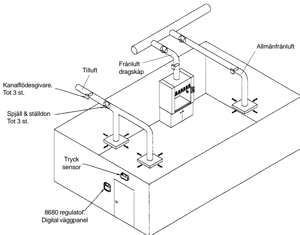
Figur 7- Exempel på laboratorieinstallation
